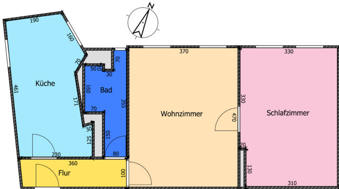
Grundriss
