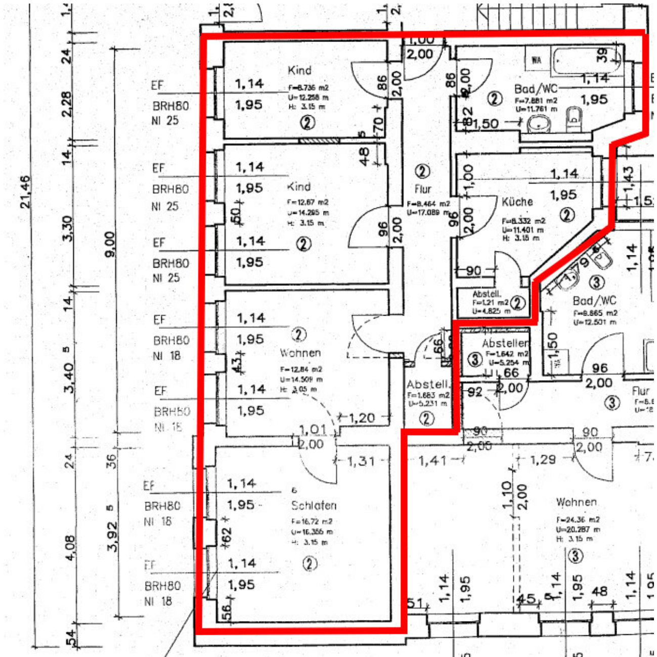
Grundriss_WE 02
