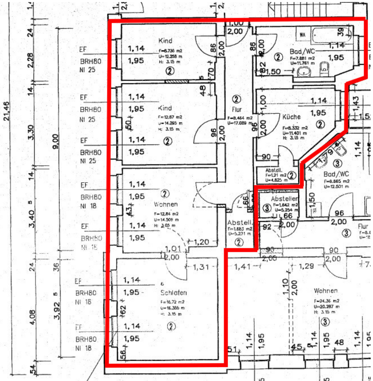
Grundriss_WE 02
