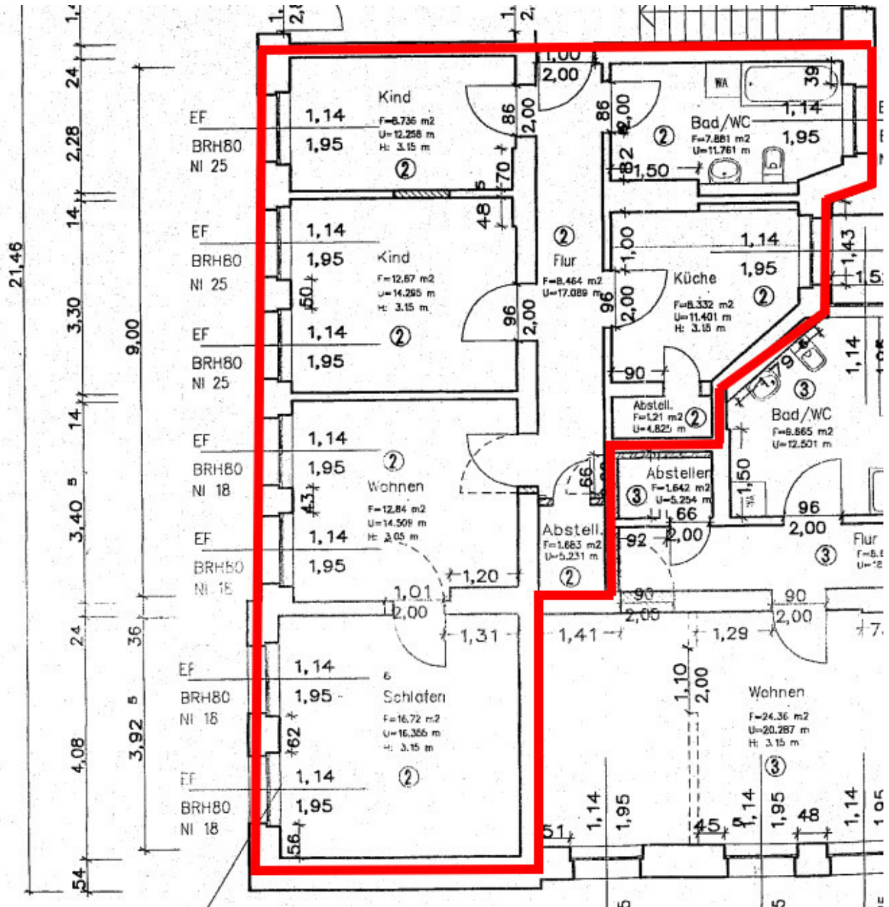
Grundriss_WE 02
