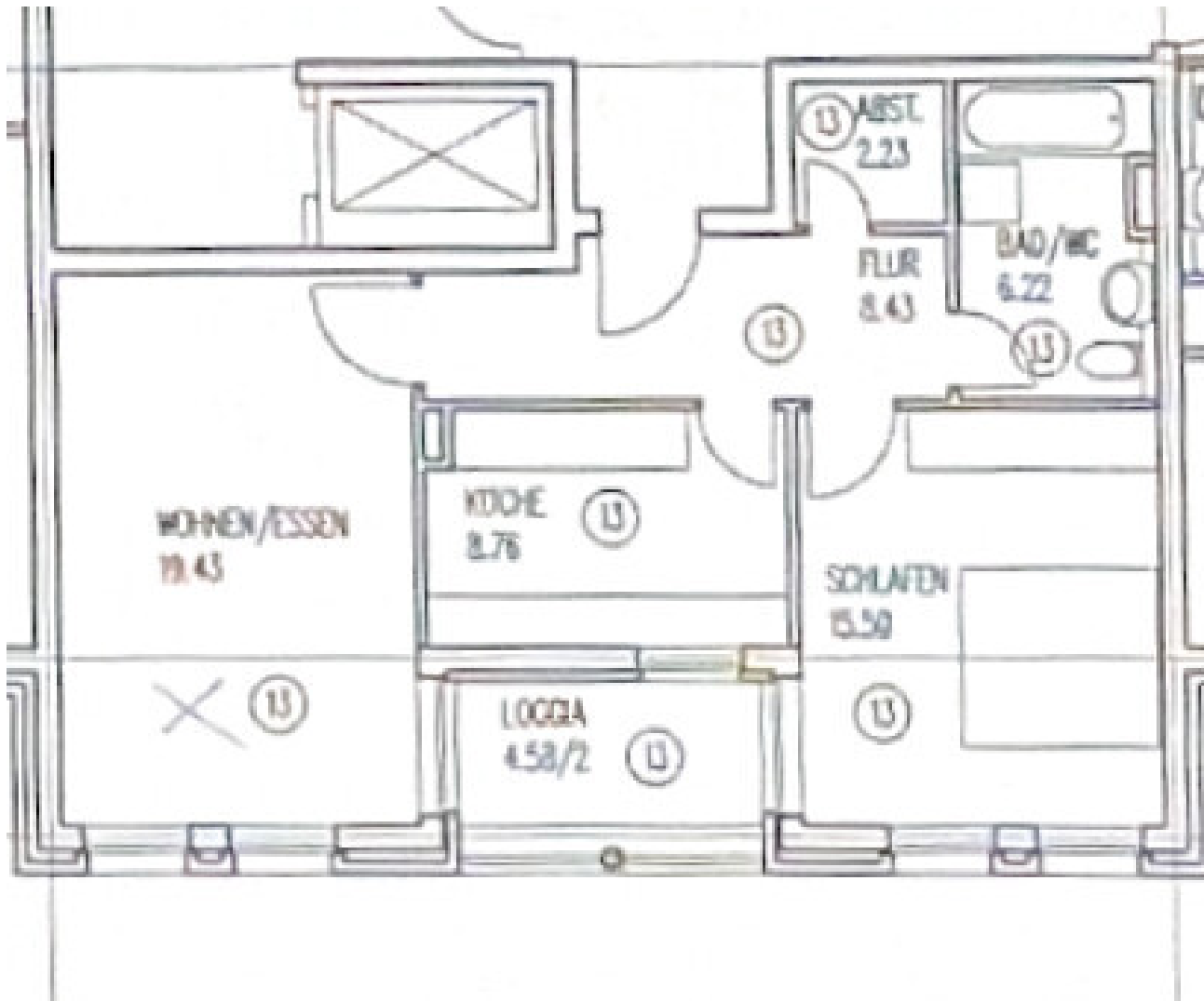
Grundriss WE13
