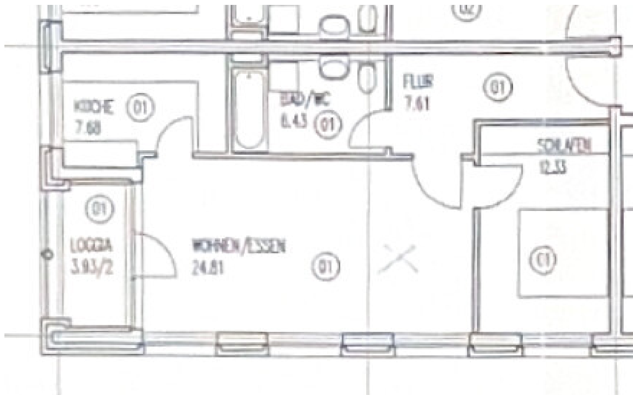
Grundriss WE01
