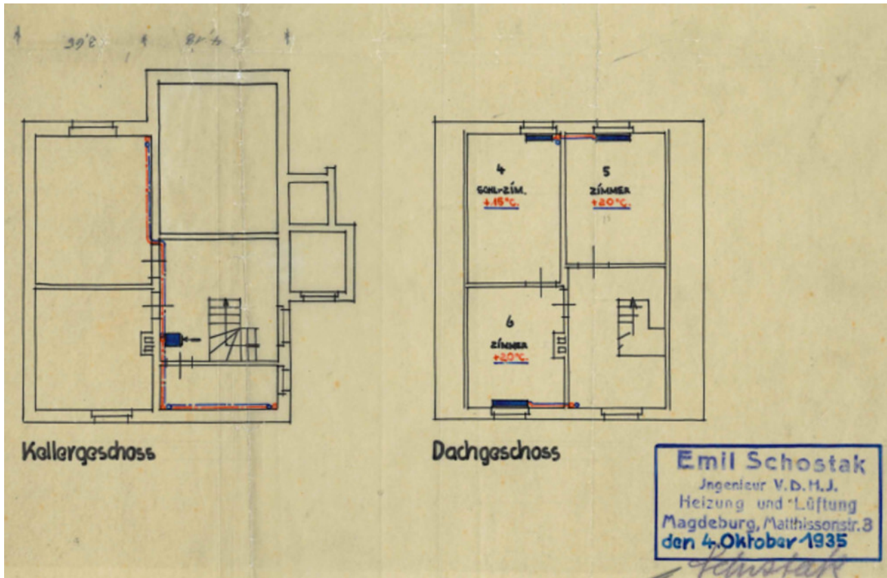
Grundriss KG, DG
