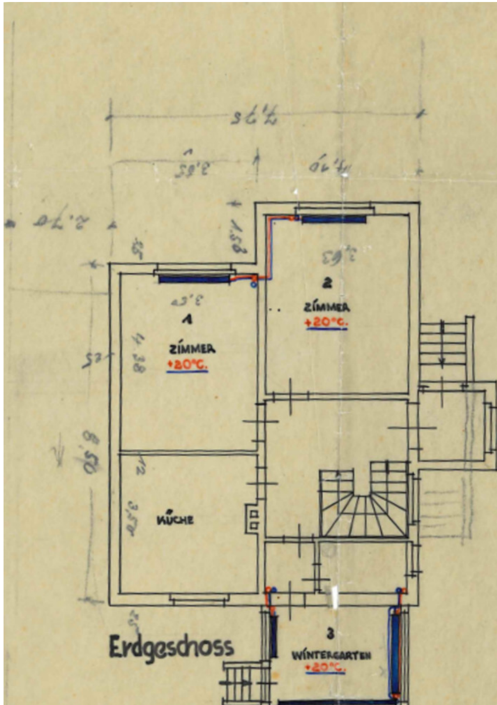
Grundriss EG
