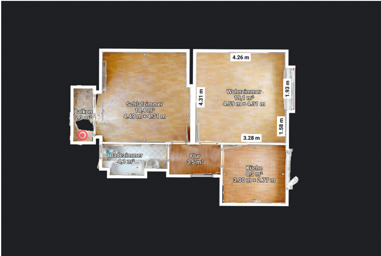
Grundriss
