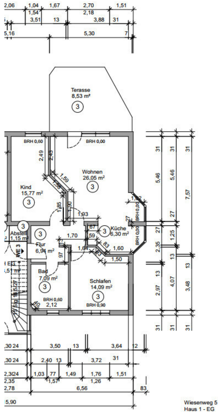
Grundriss
